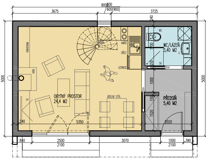
půdorys 1:100
